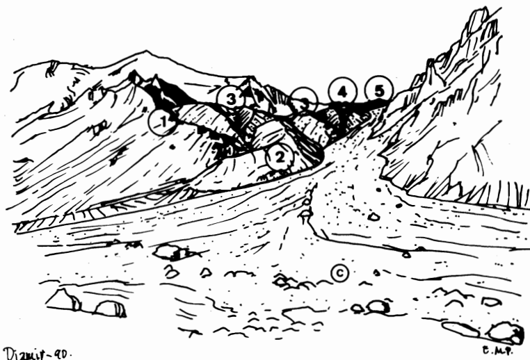
Fig. 18. Diferentes posiciones en la evolución del glaciar lateral del Paso de Diamir (Seri Galí), con su frente a 4.300 m. 1: artesa afluyente pleistocena. 2: morrena lateral de la fase intermedia. 3 y 4: dos estadios de la fase reciente. 5: posición del frente actual y salida del cono de deyección proglaciar (C).
