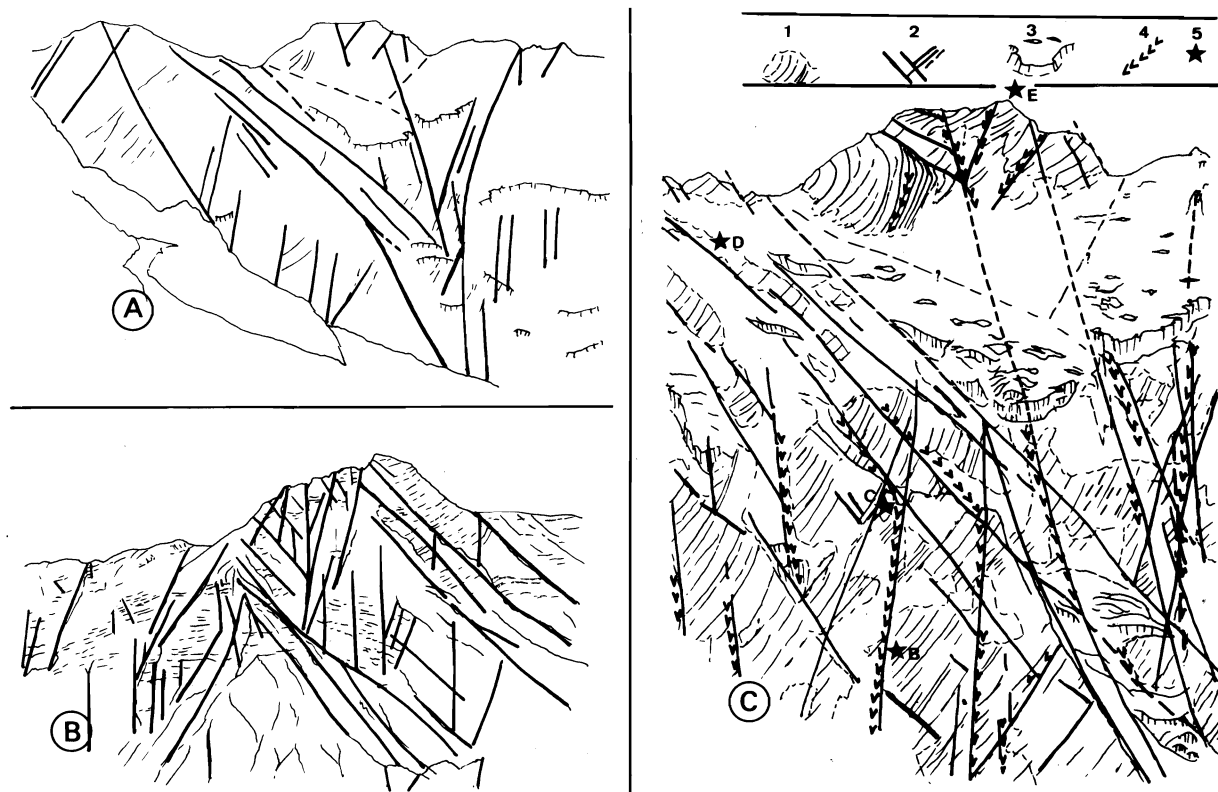
Fig. 9. Esquema morfoestructural del Nanga Parbat.
