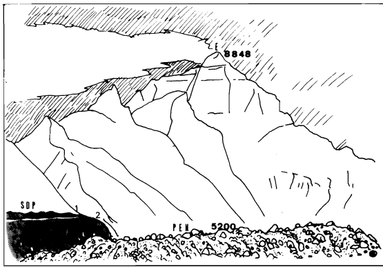
Fig. 21. Morrenas recientes en la vertiente norte del Everest.
