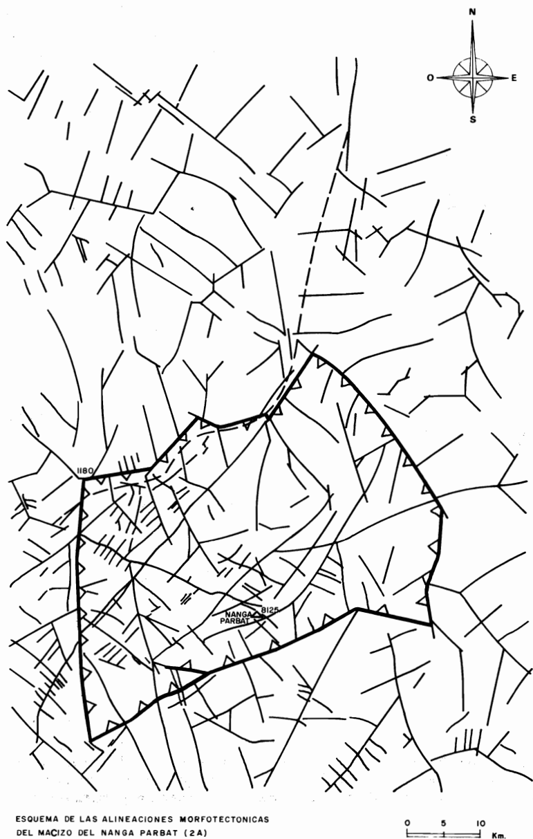
Fig. 6. Esquema de las alineaciones morfotectónicas del Macizo del Nanga Parbat (2A).
