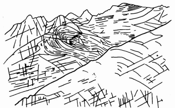
Fig. 3. Esquema de estructura plegada en el valle de Diamir.
