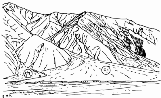
Fig. 11. Dos generaciones de conos recientes en Rupal.
