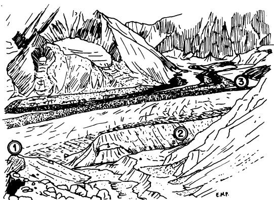
Fig. 10. Morrenas recientes y actuales de glaciar de Rupal. 1: fase intermedia. 2: PEH. 3: actuales.
