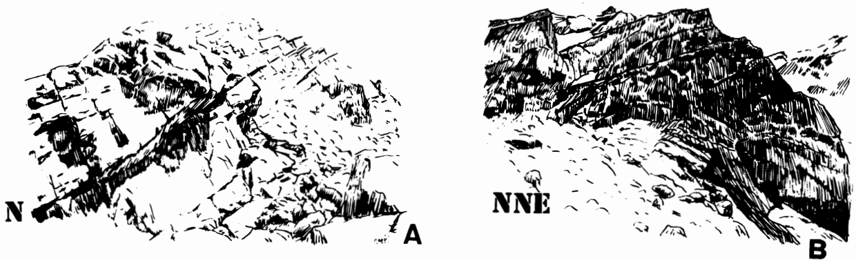
Fig. 4. Buzamiento del bandeado gneísico al Norte (A) en el alto valle de Diamir y al NNE (B), al pie de la pared de Diamir.
