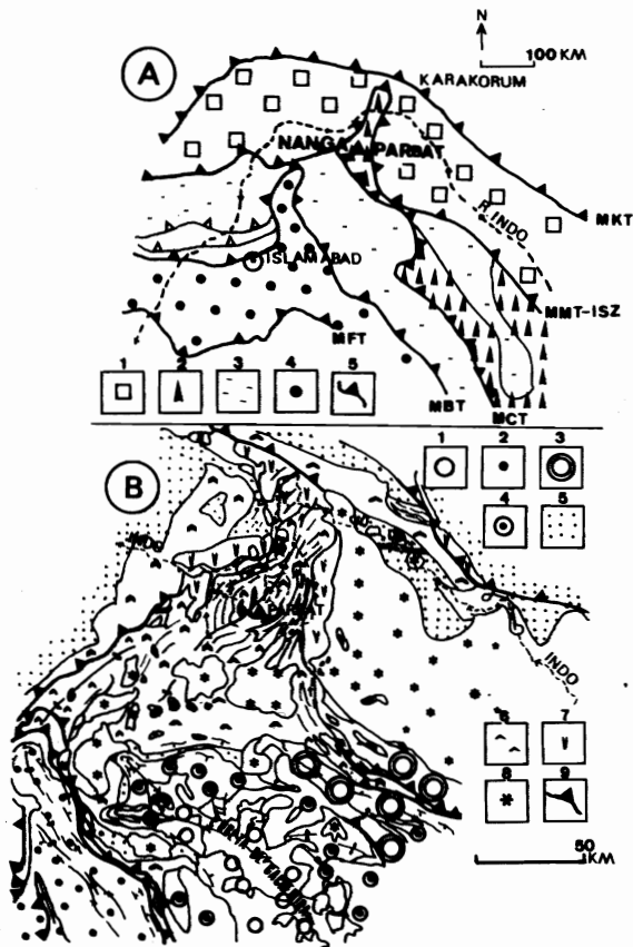
Fig. 2. EL NUDO GEOLOGICO DEL NANGA PARBAT
