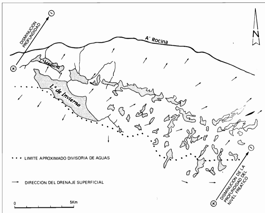
FIG. 10. En el supuesto de producirse una como la disminución del nivel freático, esta afectaría en primer lugar a la Laguna de Invierno, y seguidamente a las turbosas más meridionales (como la Laguna Mediana). Esta hipótesis coincide plenamente con los cambios detectados en la vegetación turbosa, y con la reconstrucción de la cartografía histórica de las lagunas de la Figura 7.
