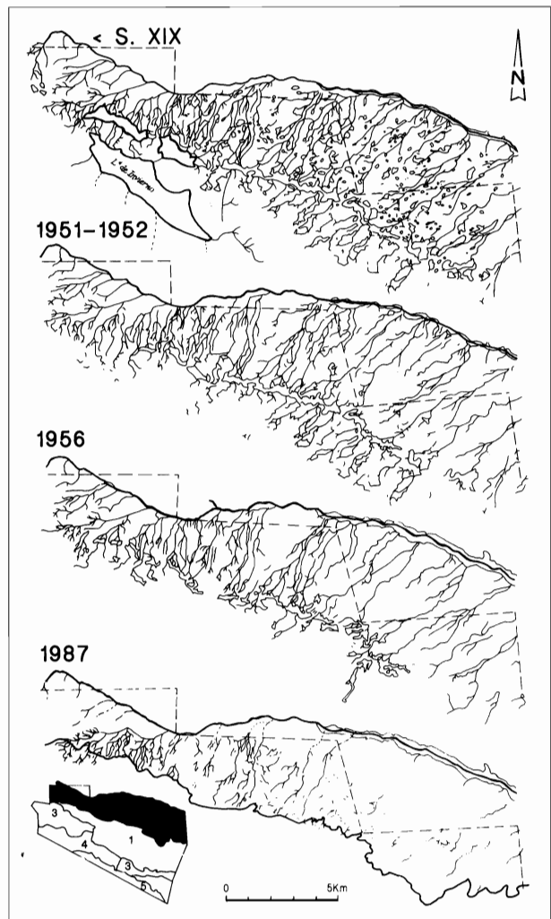
FIG. 8. Retroceso del drenaje de la Zona 2 (Cañadas) y desaparición de las pequeñas lagunas de la Zona.
