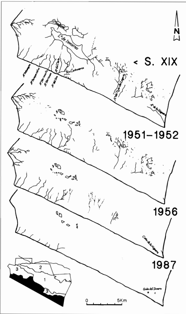
FIG. 9. Proceso de desaparición de los arroyos más orientales y pérdida de conexión del arroyo del Loro con la Laguna de Invierno.
