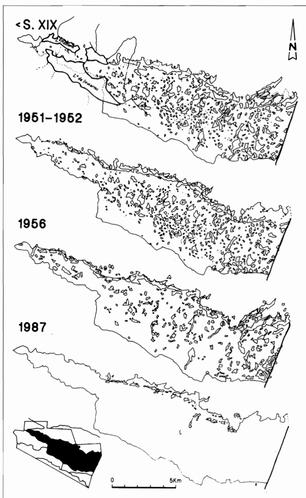
FIG. 7. Se puede observar la progresiva desaparición, de las lagunas turbosas más meridionales, desde antes del siglo XIX. Además destaca la desaparición completa de las lagunas de Invierno y La Mediana, probablemente desde finales del siglo XIX. En la cartografía se aprecia también el sentido de desaparición de las lagunas (desde SO a NE).
