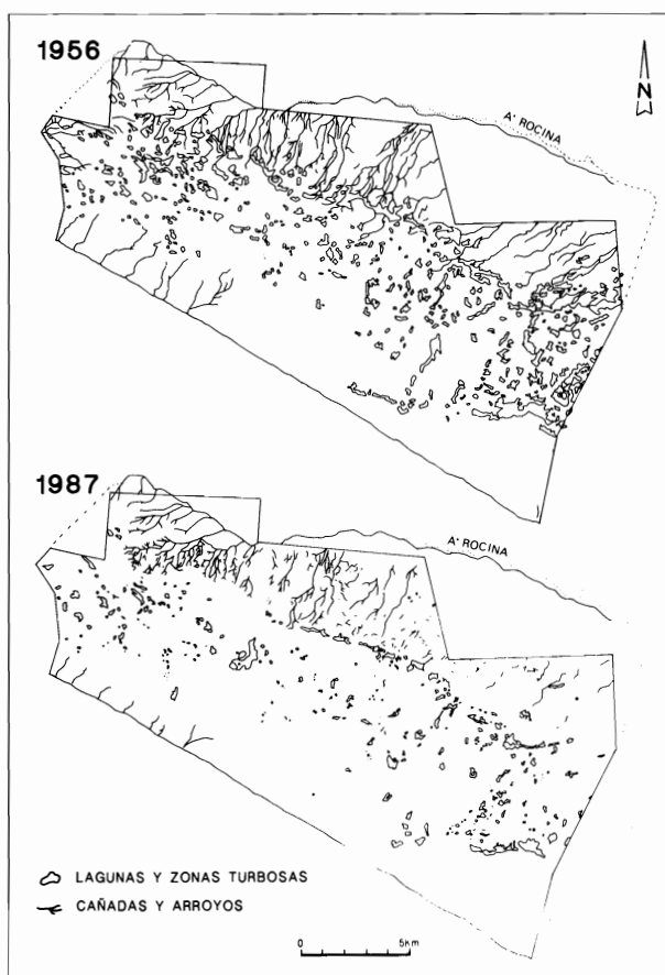
FIG. 4. Visión general de los cambios en el drenaje superficial en toda la zona de estudio, para el período 1956-1987. Se aprecia claramente la alteración del drenaje, a través de cañadas y arroyos, y la desaparición de numerosas lagunas.
