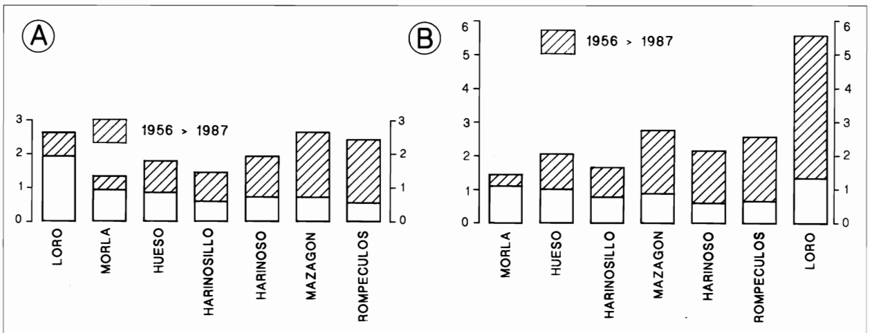
Fig. 5. Disminución de la longitud parcial (A) y total (B), de cada uno de los arroyos que conforman la Zona 4 (período 1956-1987). Globalmente la disminución ha sido superior al 60%, mientras que en la Unidad Cañadas (Zona 2), ha sido sólo del 30%.
