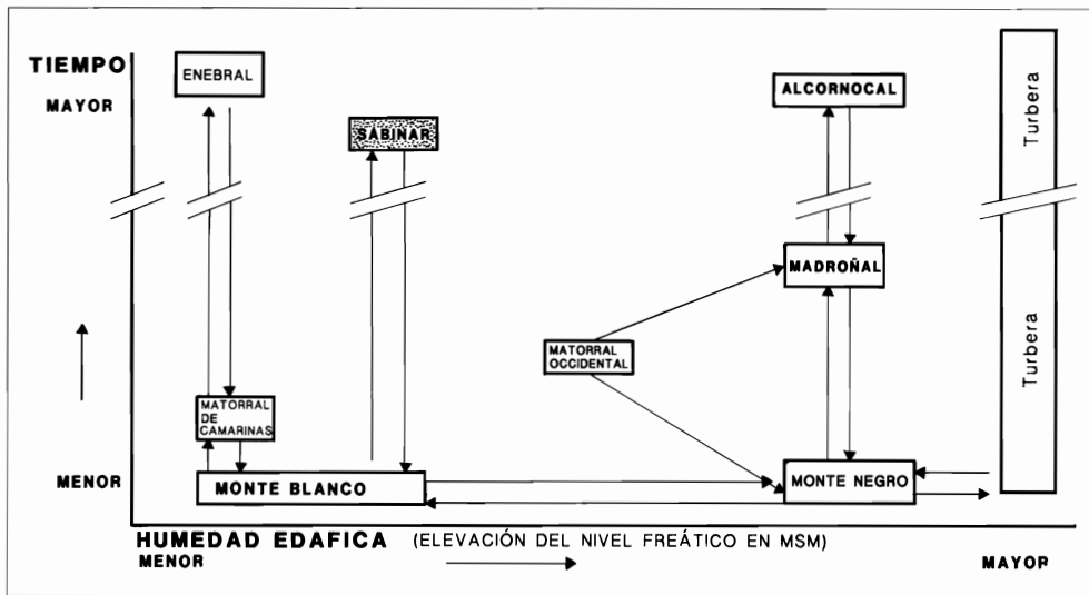
FIG. 2. Relaciones de las unidades de vegetación del Abalarío, y su evolución en función del tiempo (sucesión), y de la humedad edáfica. Fuente: elaboración propia.
