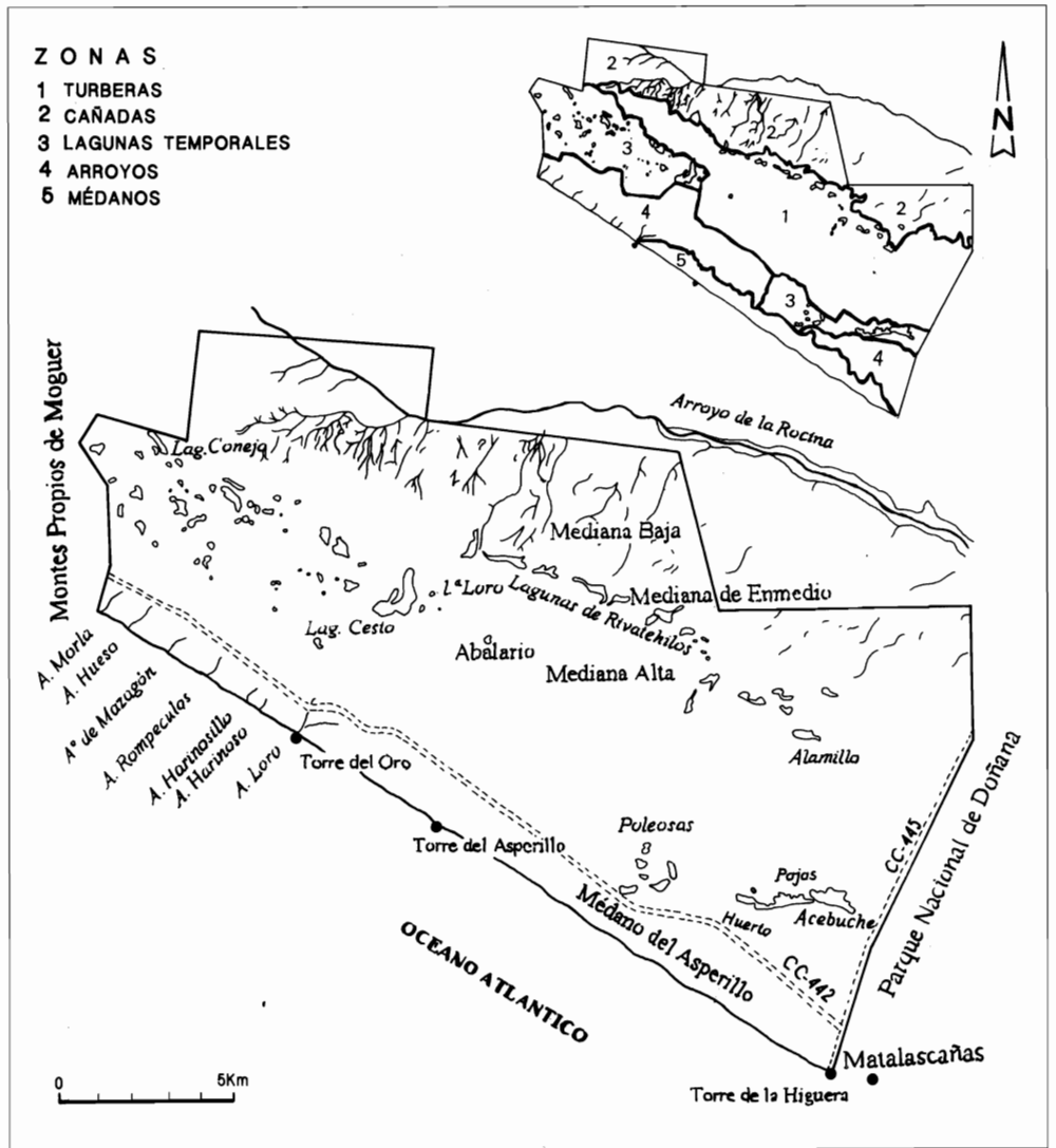
FIG. 3. (arriba) División de la zona de estudio en función de las diferentes características del avenamiento y la vegetación; (abajo) Mapa actual del área de trabajo con las principales localidades, lagunas, arroyos y otros topónimos.
