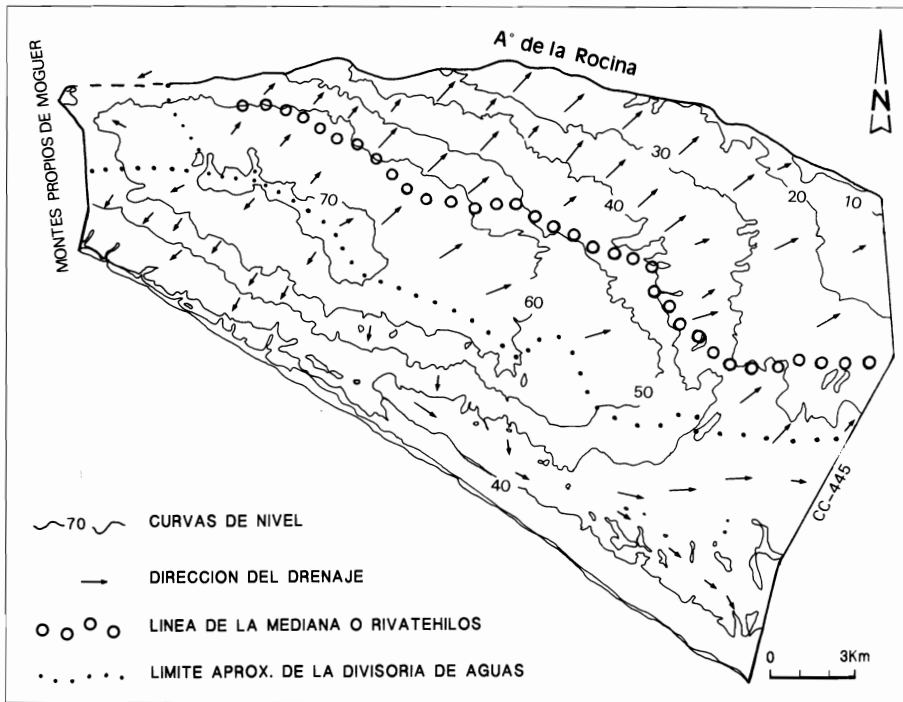
FIG. 6. Mapa altitudinal de la zona de trabajo, con la reconstrucción de la línea de cauce que ocuparía un hipotético desagüe, del que las lagunas de Rivatehilos serían su testigo. Se aprecia claramente que la topografía obliga a que la escorrentía se organice hacia el Arroyo de la Rocina, y no en dirección al supuesto cauce desaparecido. Fuente: basado en GONZALO Y TARÍN (1887), ESPINA - ESTÉVEZ (1992), y modificado por los autores en base al M.T.N. y a un vuelo de 1956.
