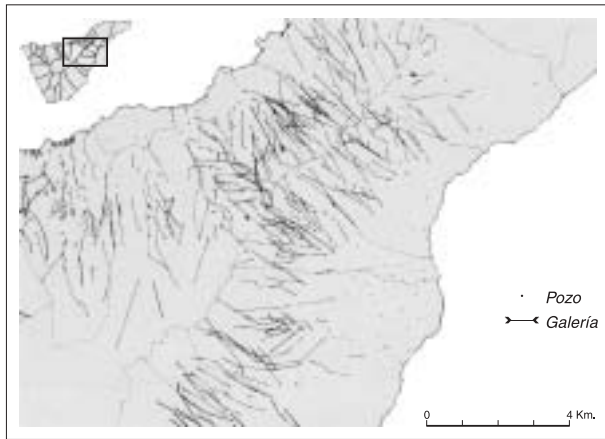
FIG. 7. Galerías y pozos en la dorsal de Tenerife. Fuente: Geografía de Canarias , 1993, vol. I, pág. 137.
