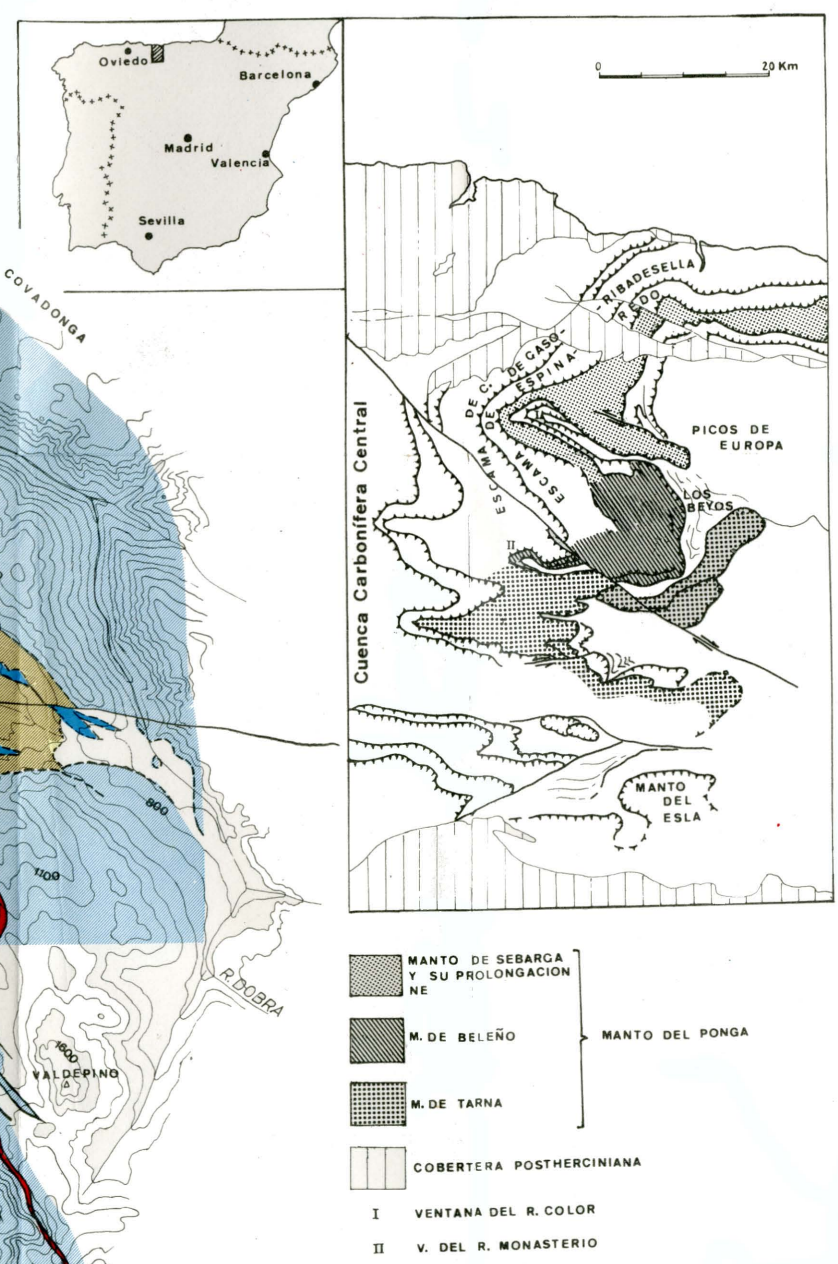
Situación de la región estudiada y esquema tectónico general del manto de Ponga
