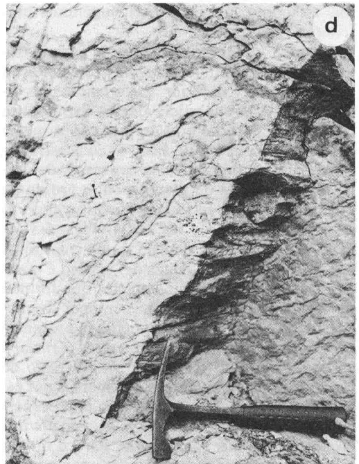
Fig. 7.—a: Taphrhelminthopsis (L-4 en Fig. 5). b: Cruziana goldfussi (L-3 en Fig. 5). c: Laminación cruzada en cuarcitas del tramo inferior de las Cuarcitas y Filitas del Invernadeiro. d: Capas con Dictyodora . Obsérvense las formas en «tronco de cono», en la sección normal al plano de estratificación (L-7 en Fig. 5).
