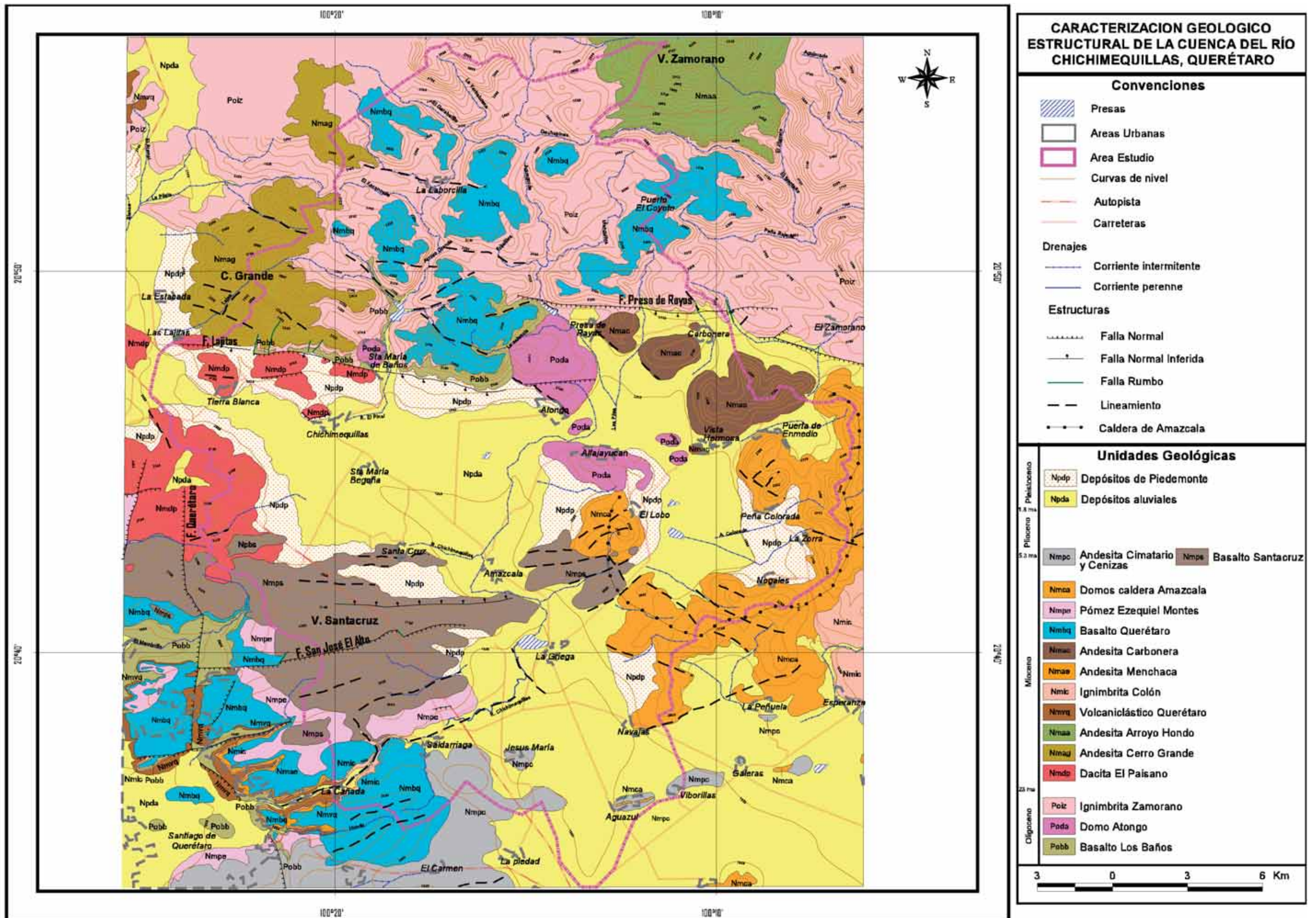
Figura 2. Mapa Geológico-Estructural de la cuenca del río Chichimequillas.
