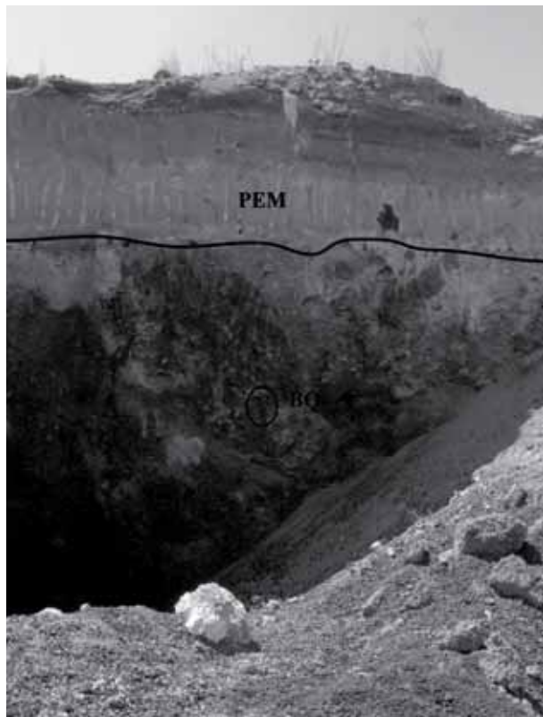
Figura 5. Pómez Ezequiel Montes (PEM), sobreyaciendo al Basalto Querétaro (BQ), al sur de la localidad de Saldarriaga. La escala (martillo) se encuentra al lado izquierdo de la sigla BQ, dentro del círculo negro.
