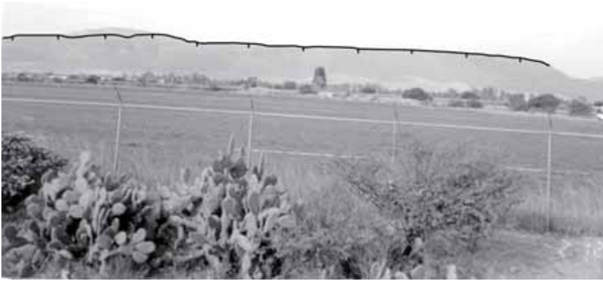
Figura 8. Vista de un escarpe característico de la Falla Lajitas en el tramo comprendido entre las poblaciones de Santa María de los Baños y Atongo.
