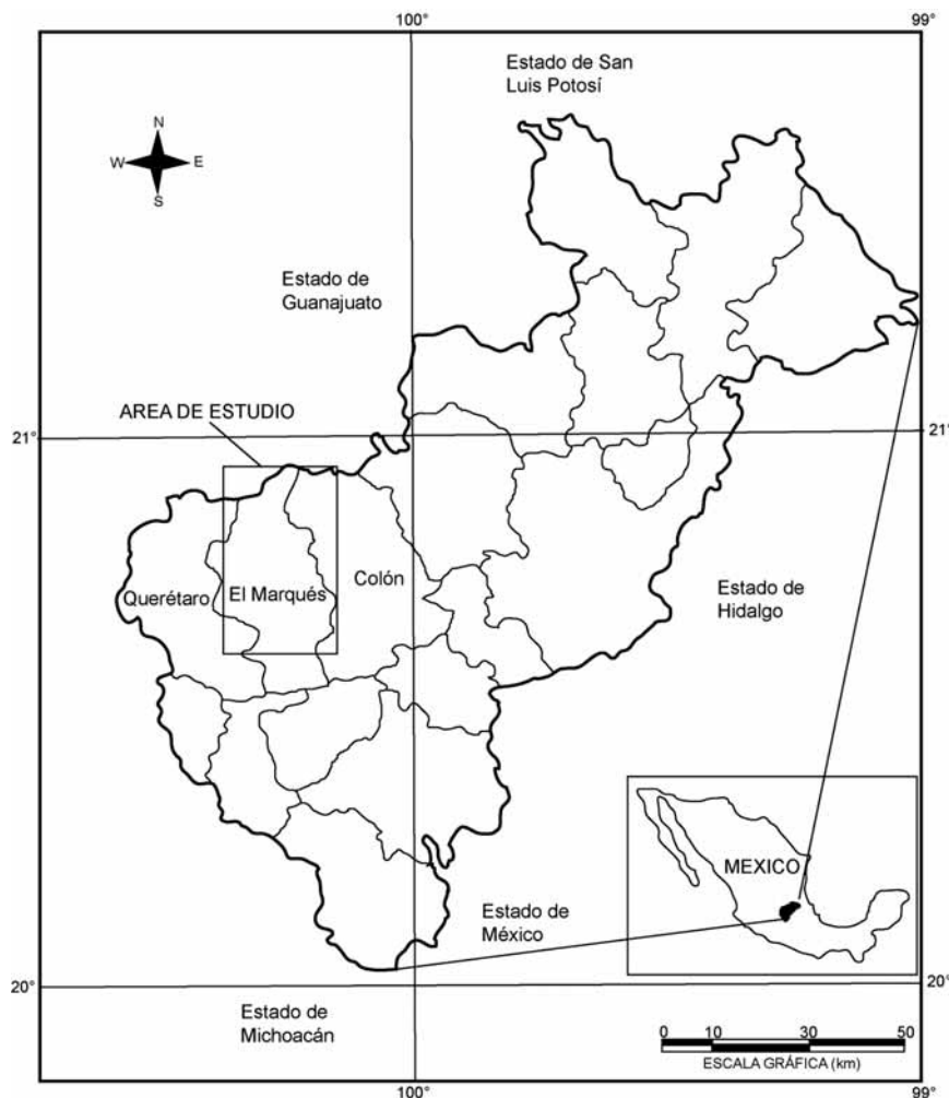
Figura 1. Localización de la zona de estudio dentro del estado de Querétaro.
